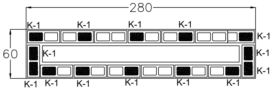
ESTRUCTURA DE PÓRTICO PR-04 PLANTA
