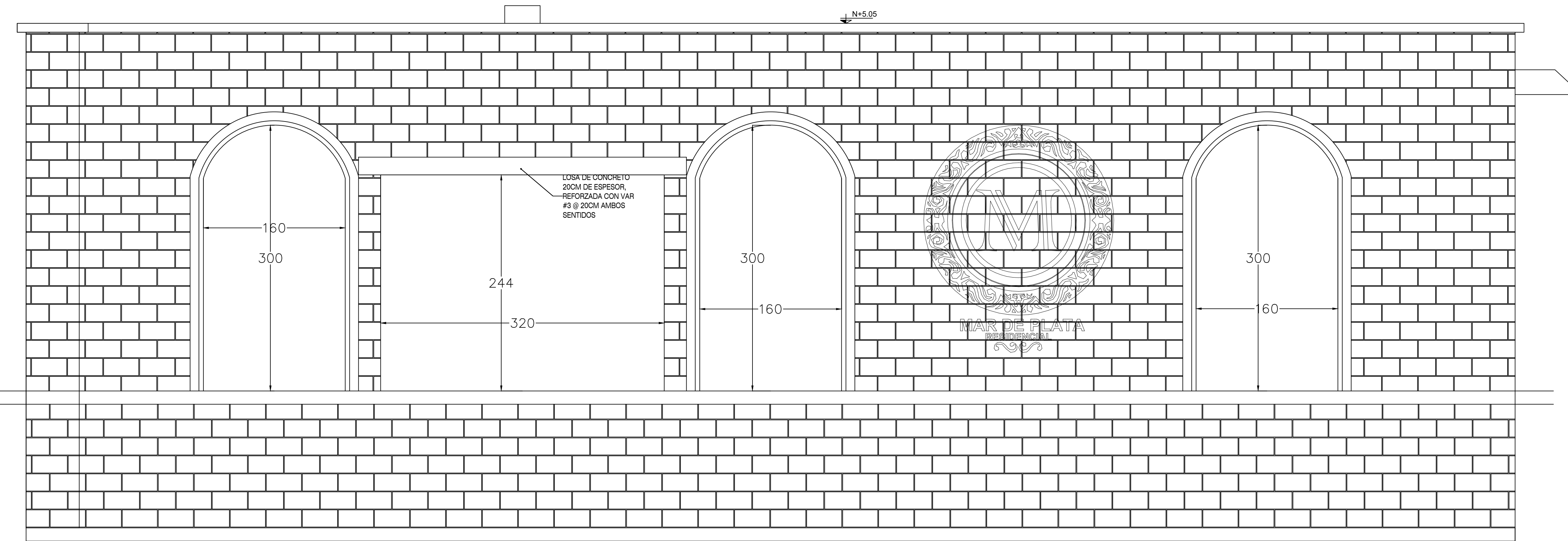
ESTRUCTURA DE PÓRTICO PR-02 ALZADO
