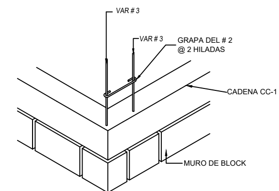
DETALLE DE ANCLAJE DE CASTILLO EN ESQUINA O INTERSECCIÓN ISOMETRICO-ESCALA 1:20
