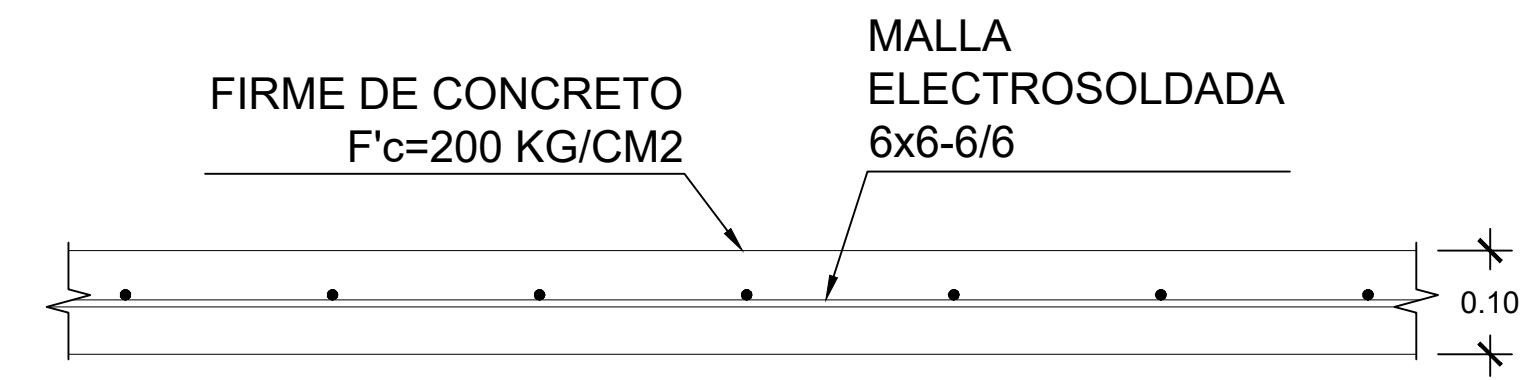
ARMADO DE FIRME DE CONCRETO ALZADO ESCALA 1:10
