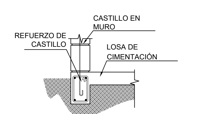
ANCLAJE DE REFUERZO DE MUROS ALZADO
