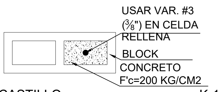
CASTILLO PLANTA ESC. 1:10
