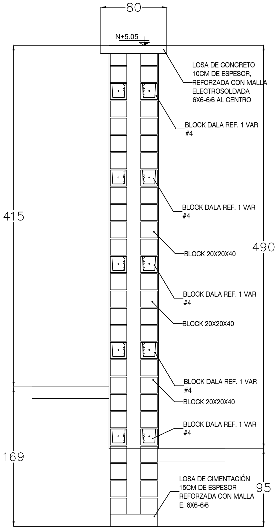
CORTE ESTRUCTURA DE PÓRTICO PR-02, PR-03 Y PR-04 ALZADO
