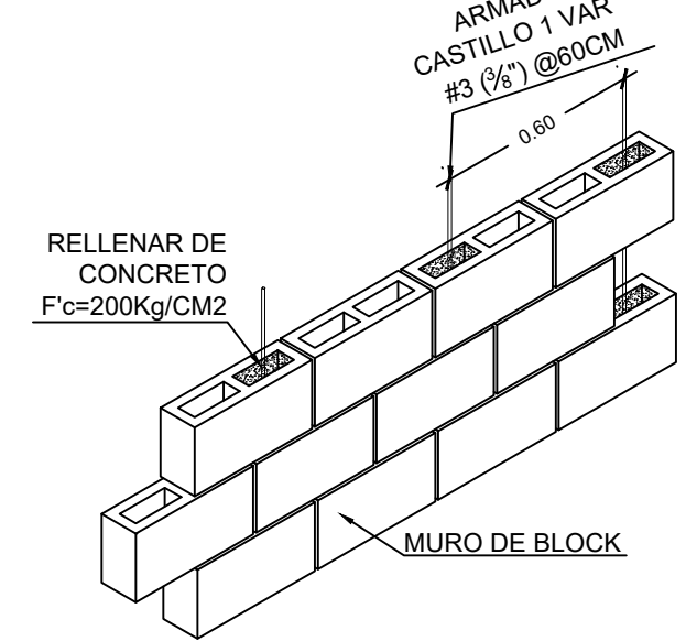
DETALLE TIPO DE REFUERZO PARA MURO DE BLOCK ISOMETRICO ESCALA 1:20
